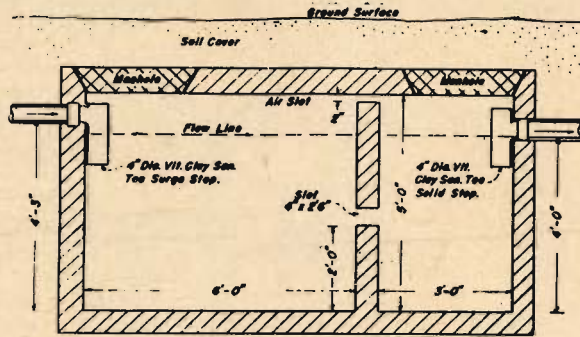
LONGITUDINAL SECTION A-A
